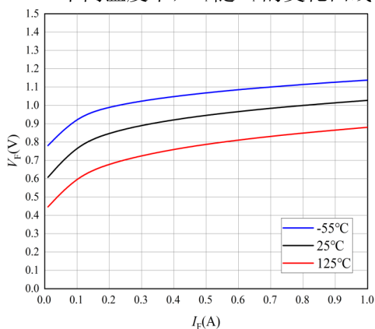
图 1 正向特性曲线
