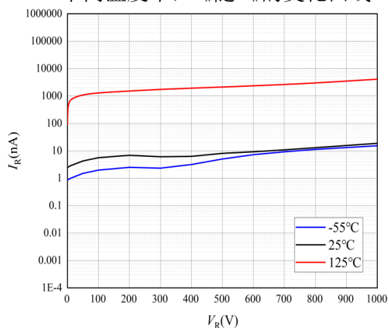
图 2 反向特性曲线
