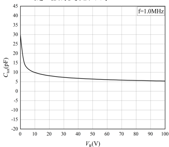
图 3 结电容特性曲线
