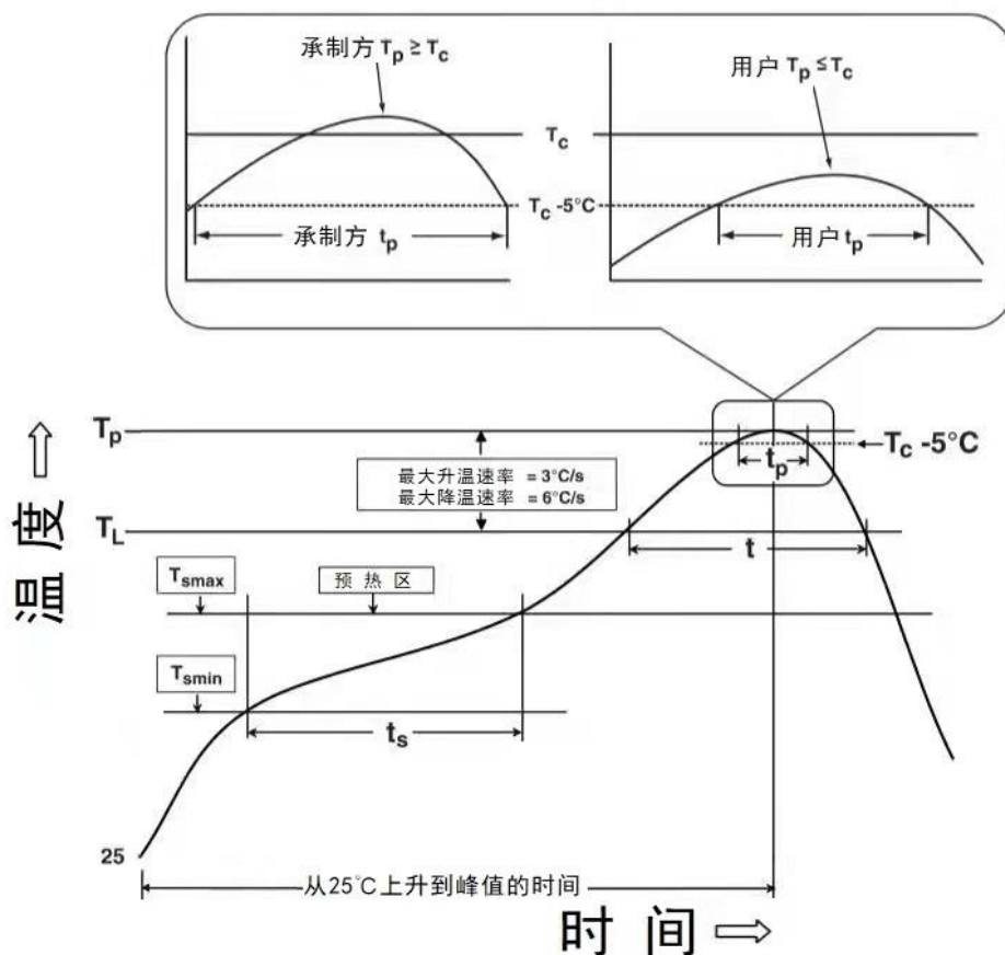
图 17 回流温度-时间分布图
