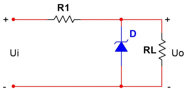
图 16 典型的应用连接图
