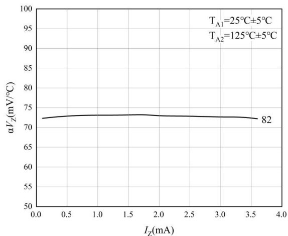
图 14 温度漂移特性曲线-4
