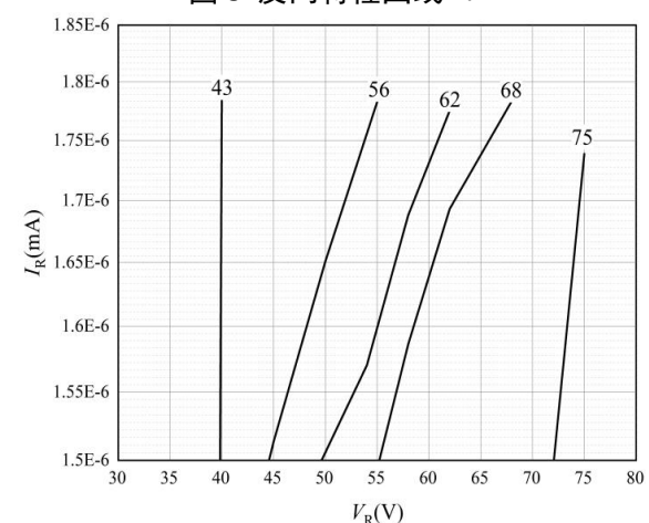
图 10 反向特性曲线-6
