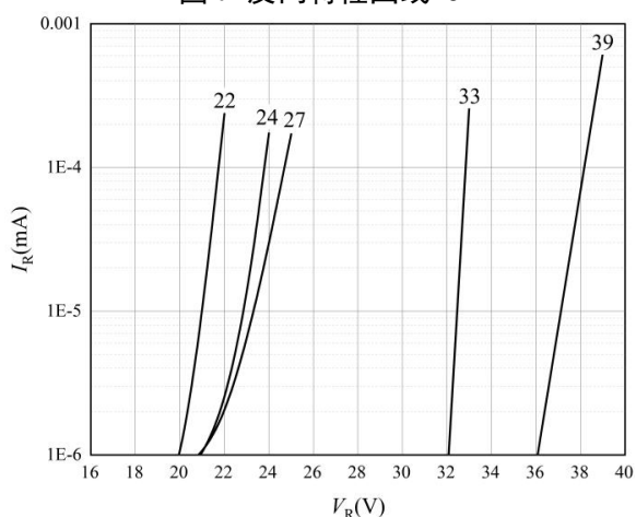
图 9 反向特性曲线-5
