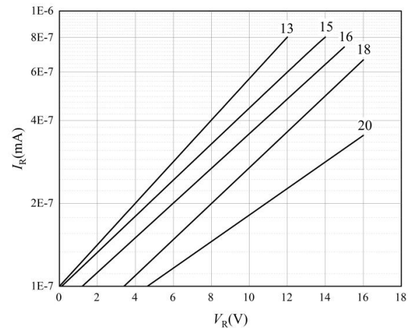
图 8 反向特性曲线-4
