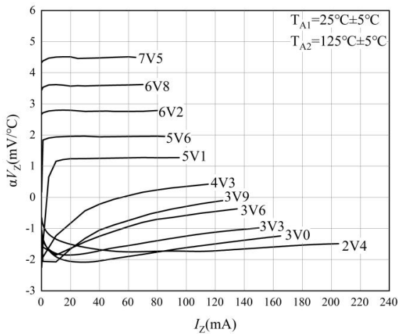
图 11 温度漂移特性曲线-1
