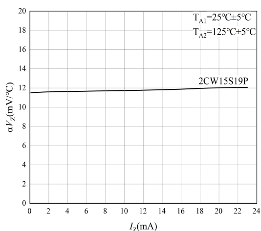
图 3 温度漂移特性曲线
