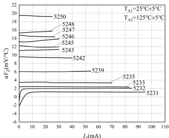
图 8 温度漂移特性曲线
