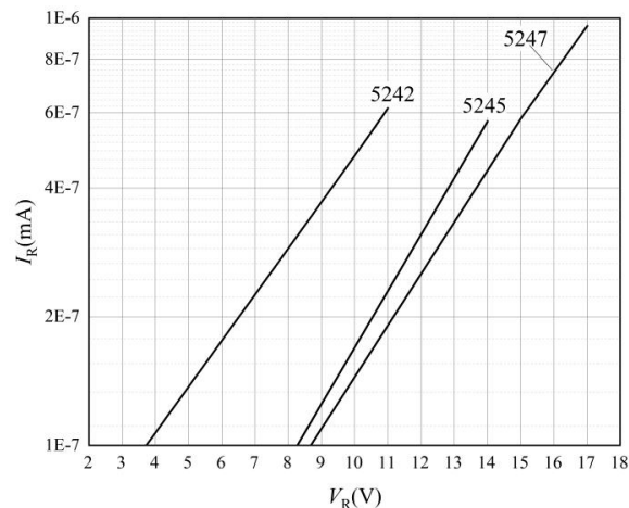
图 6 反向特性曲线-4
