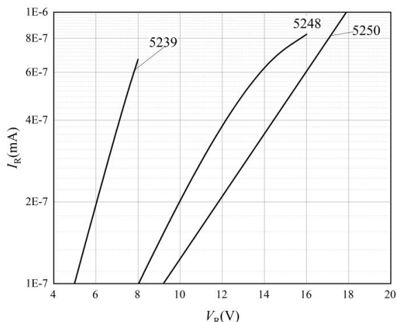
图 5 反向特性曲线-3
