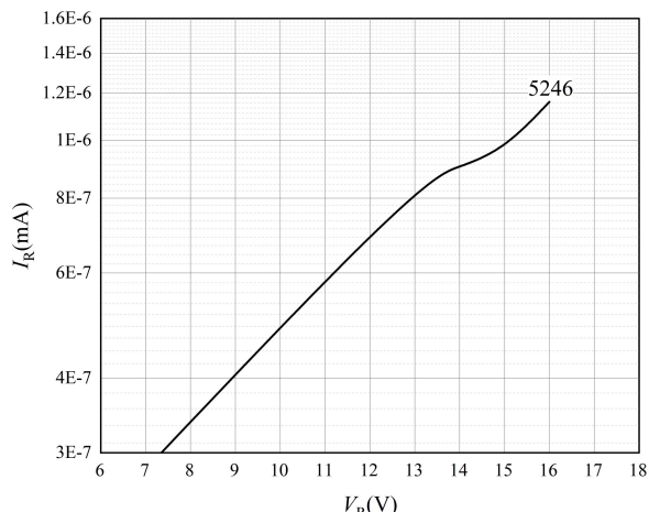
图 7 反向特性曲线-5
