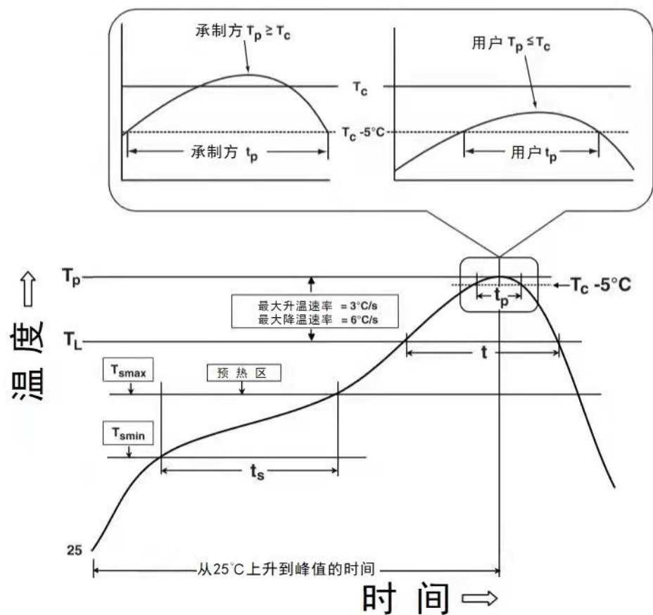
图 11 回流温度-时间分布图
