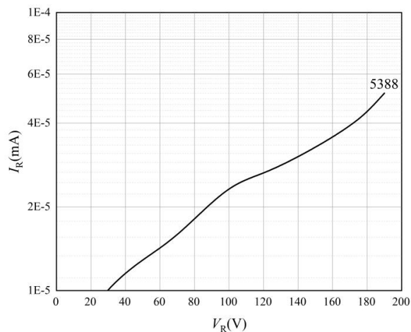
图 5 反向特性曲线-3
