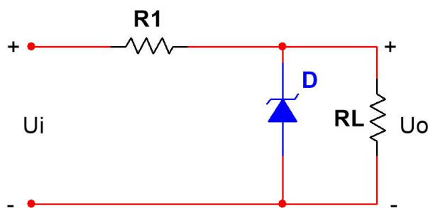
图 10 典型的应用连接图
