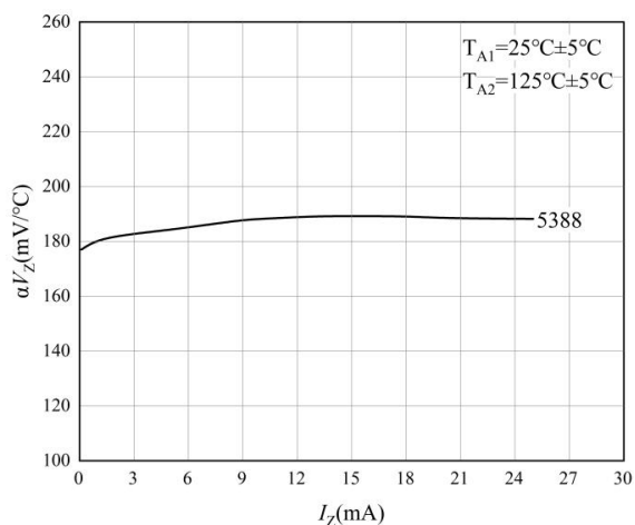
图 8 温度漂移特性曲线-3
