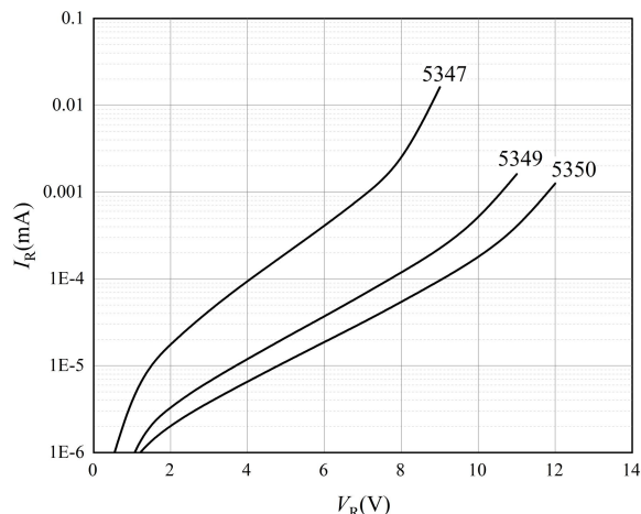
图 3 反向特性曲线-1
