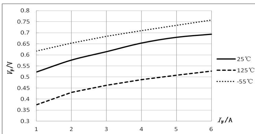
图2 V_F-I_F 特性曲线
