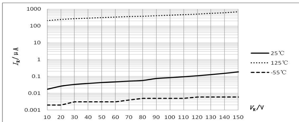
图 1 I_R - V_R 特性曲线
