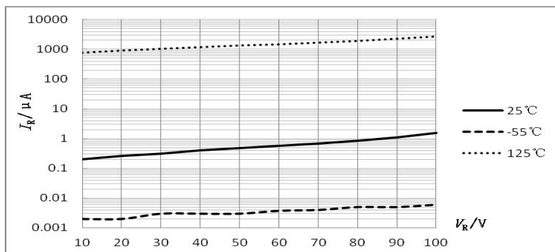
图1 I_R - V_R 特性曲线
