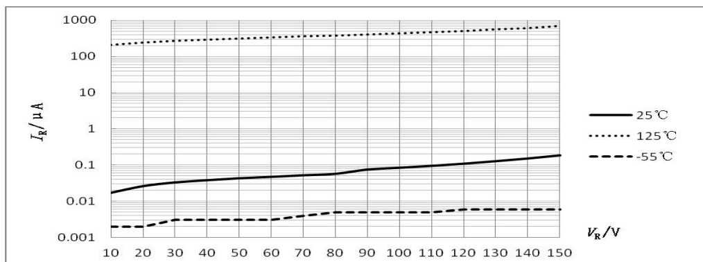
图 1 I_R - V_R 特性曲线
