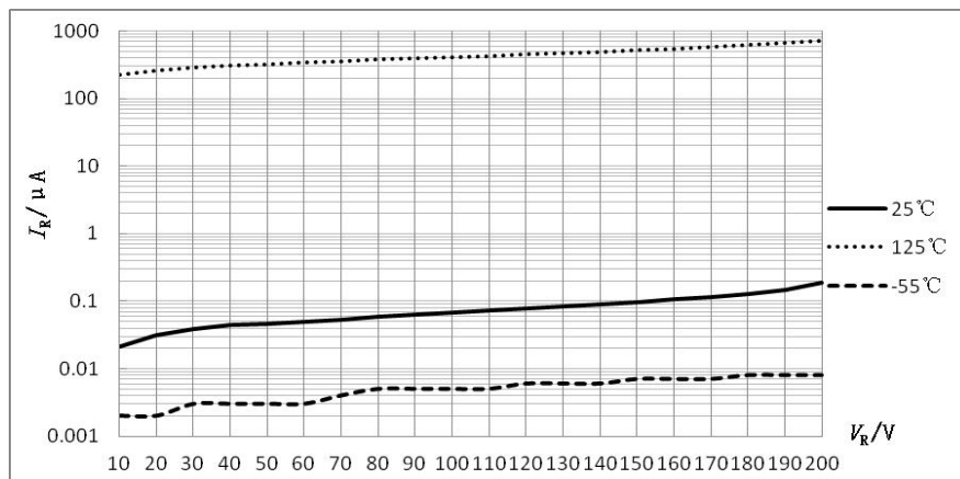
图1 I_R-V_R 特性曲线
