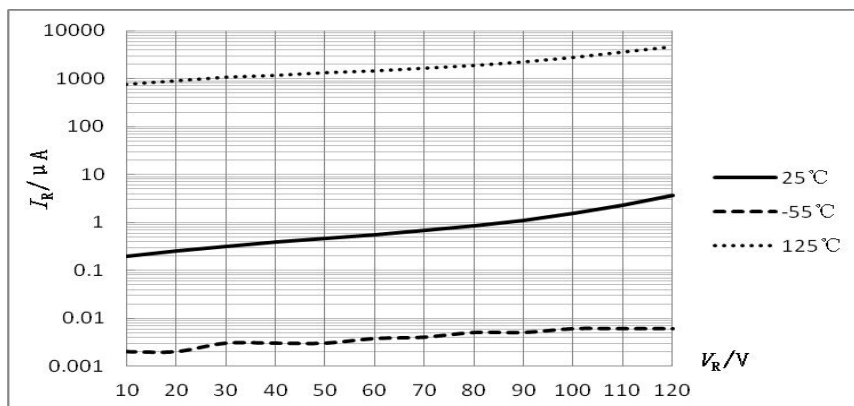
图1 I_R — V_R 特性曲线
