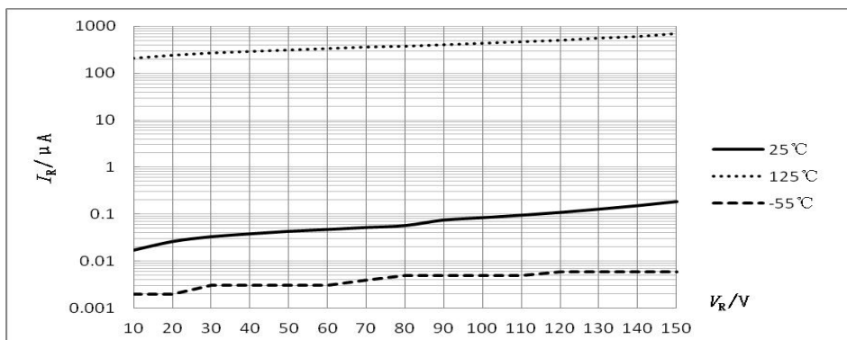
图1 I_R-V_R 特性曲线
