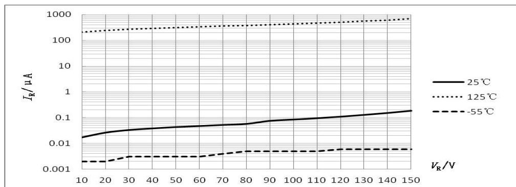
图1 I_R — V_R 特性曲线
