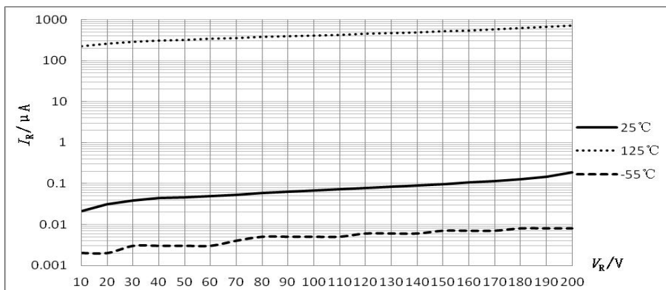
图1 I_R - V_R 特性曲线
