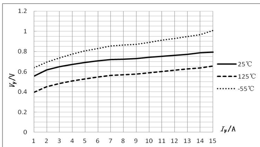
图2 V_F - I_F 特性曲线
