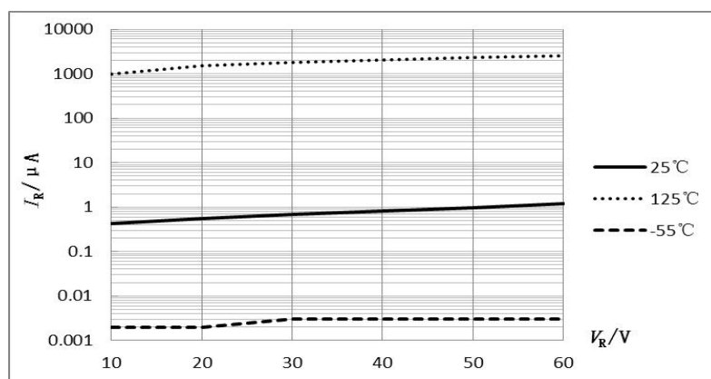
图1 I_R - V_R 特性曲线
