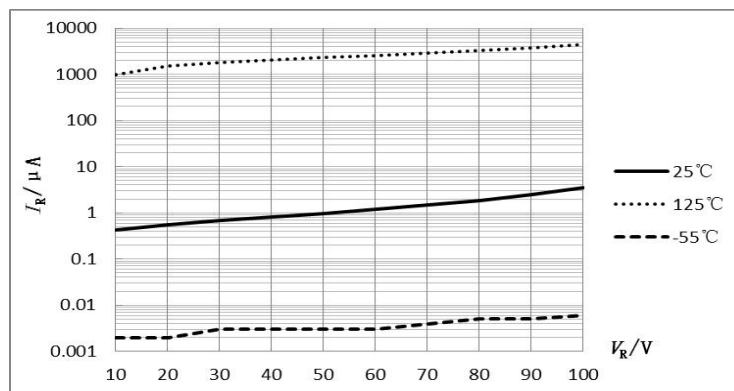
图 1 I_R - V_R 特性曲线
