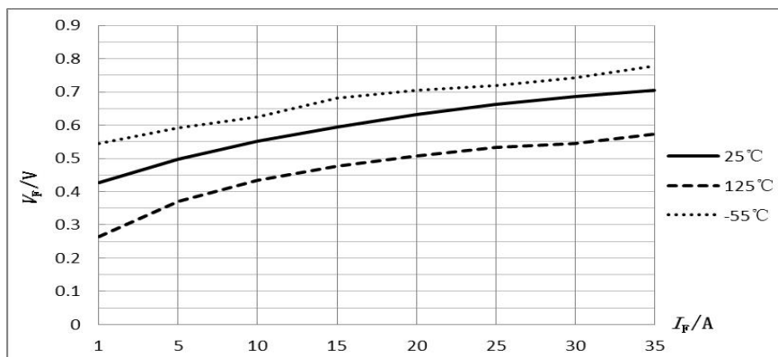
图2 V_F - I_F 特性曲线
