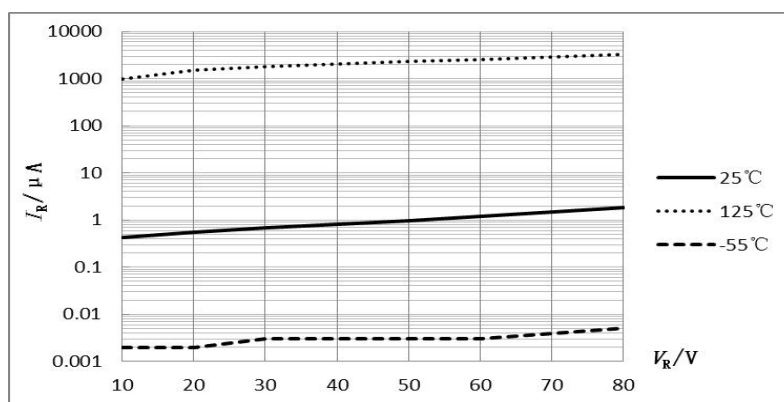
图 1 I_R - V_R 特性曲线
