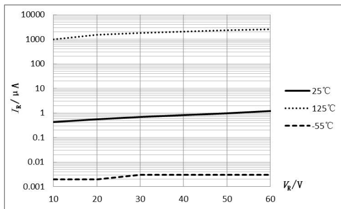
图 1 I_R - V_R 特性曲线
