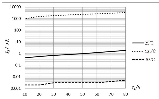
图 1 I_R - V_R 特性曲线
