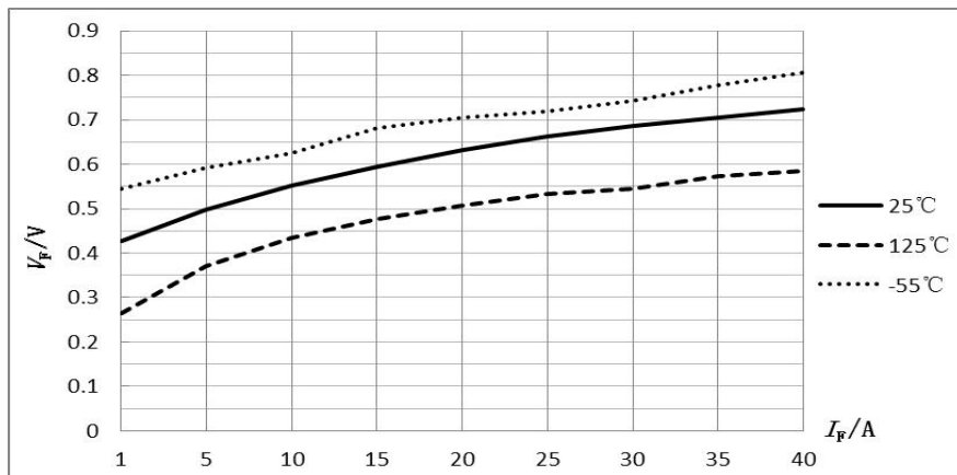
图 2 V_F — I_F 特性曲线
