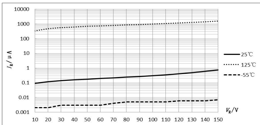
图 1 I_R - V_R 特性曲线
