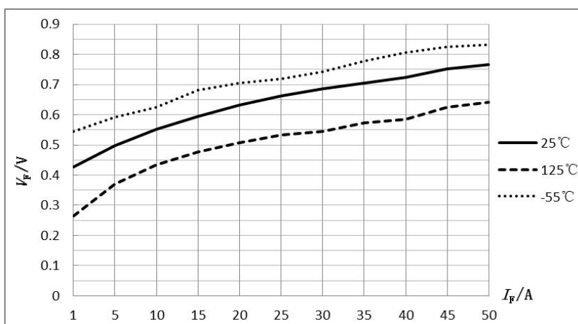
图 2 V_F - I_F 特性曲线
