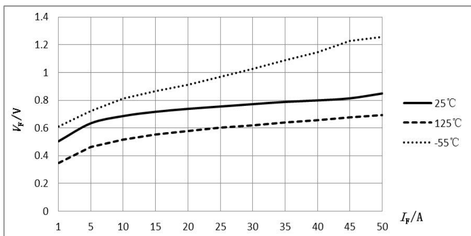
图 2 V_F — I_F 特性曲线
