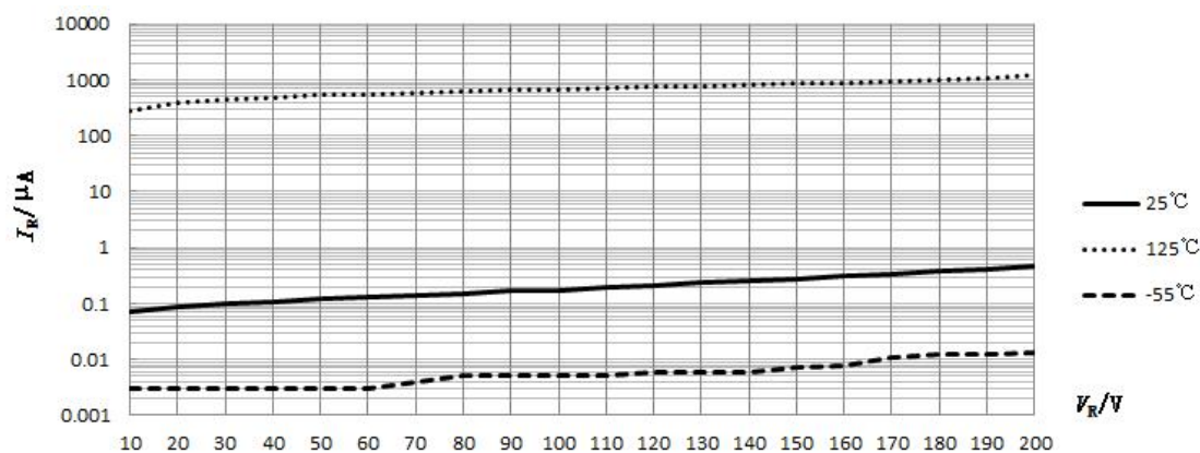
图 1 I_R — V_R 特性曲线
