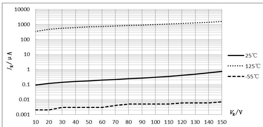
图 1 I_R - V_R 特性曲线
