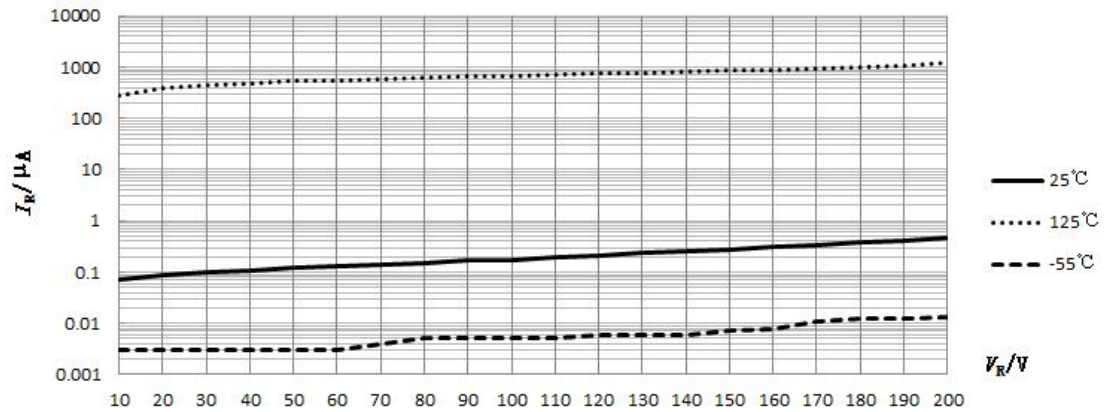
图1 I_R — V_R 特性曲线
