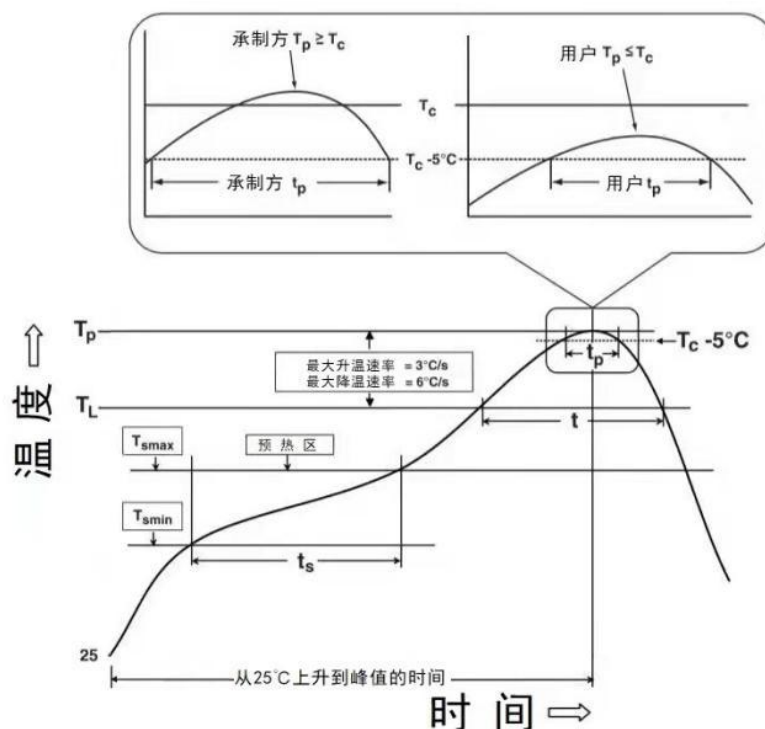
图 6 回流温度-时间分布图
