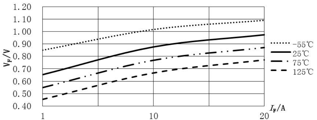
图 2 I_F-V_F 特性曲线
