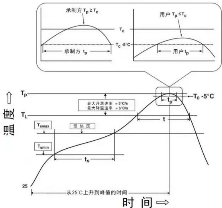
图 6 回流温度-时间分布图
