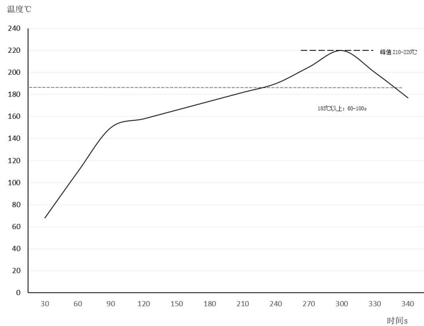
图 8 建议的回流焊曲线
