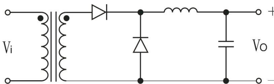
图 6 整流加续流电路
