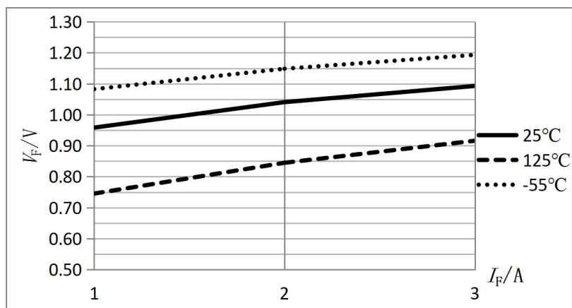
图2 V_F — I_F 特性曲线
