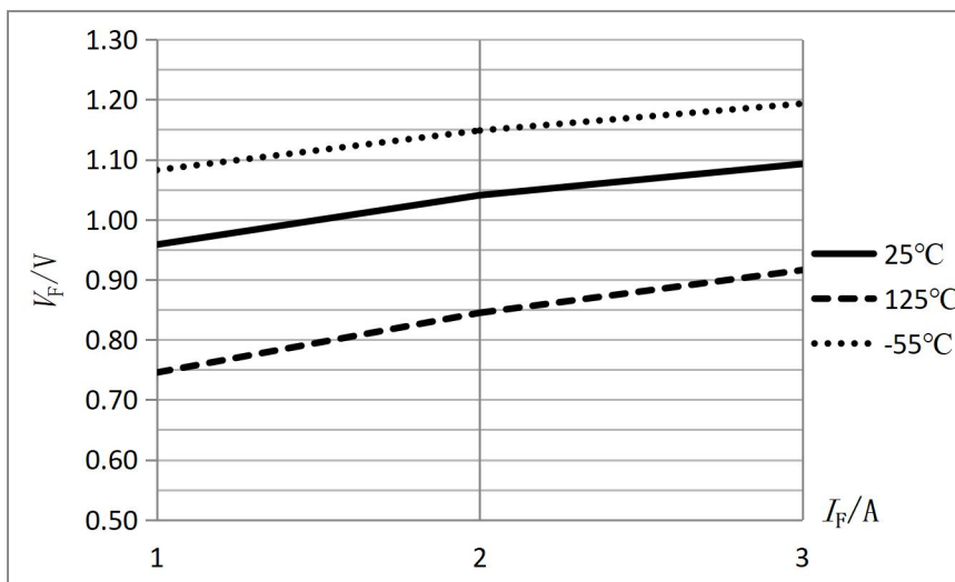
图2 V_F - I_F 特性曲线
