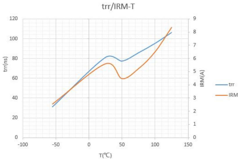
图 3 t_{rr}/I_{RM} -T 特性曲线
