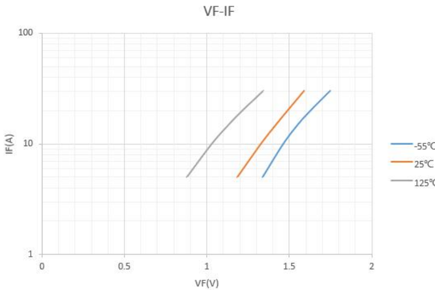
图 2 V_F-I_F 特性曲线
