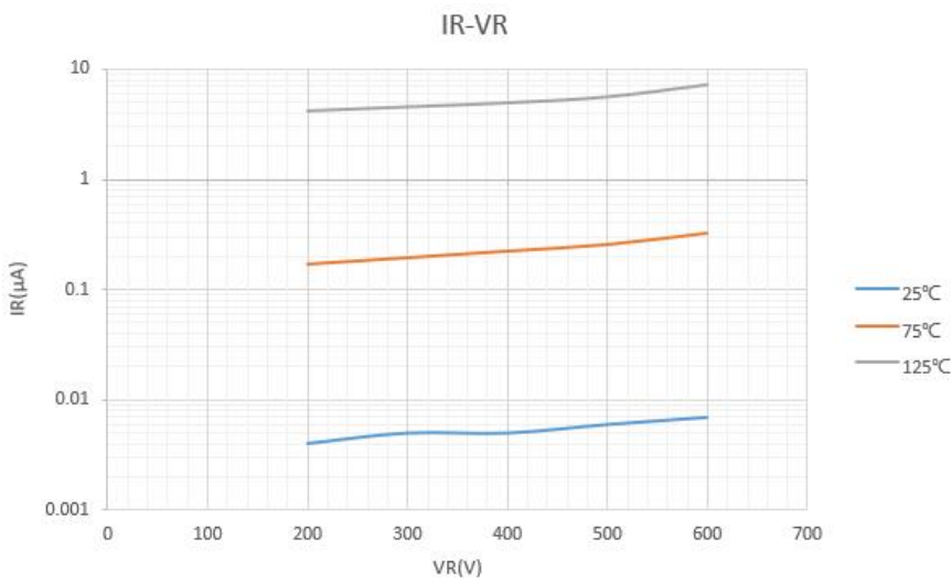
图 1 I_R-V_R 特性曲线
