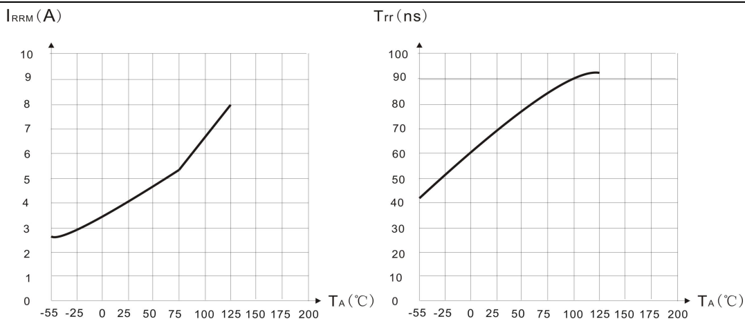
图 3 t_{rr}/I_{RM} -T 特性曲线
