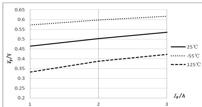
图2 V_F - I_F 特性曲线
