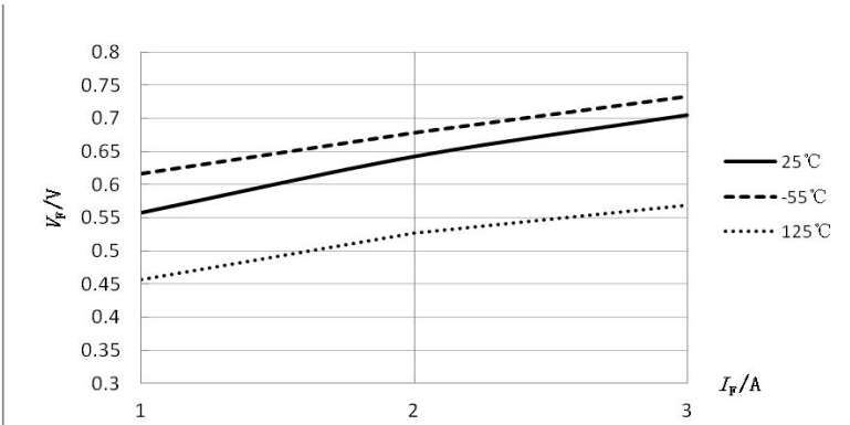
图 2 V_F — I_F 特性曲线
