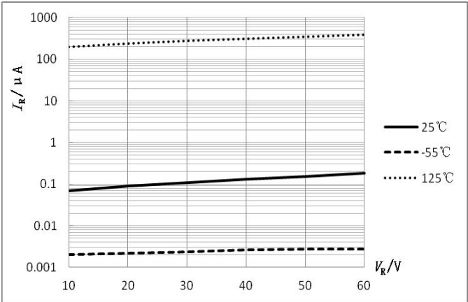
图 1 I_R — V_R 特性曲线
