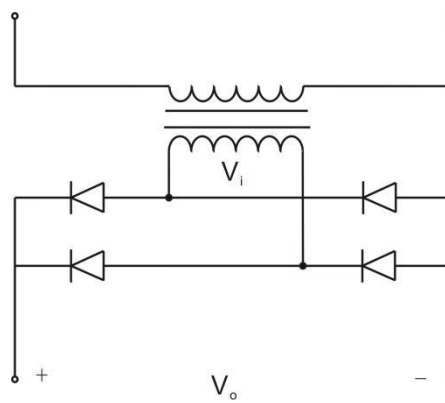
图 5 单相全波整流电路
