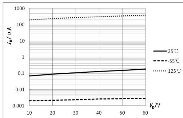
图 1 I_R - V_R 特性曲线
