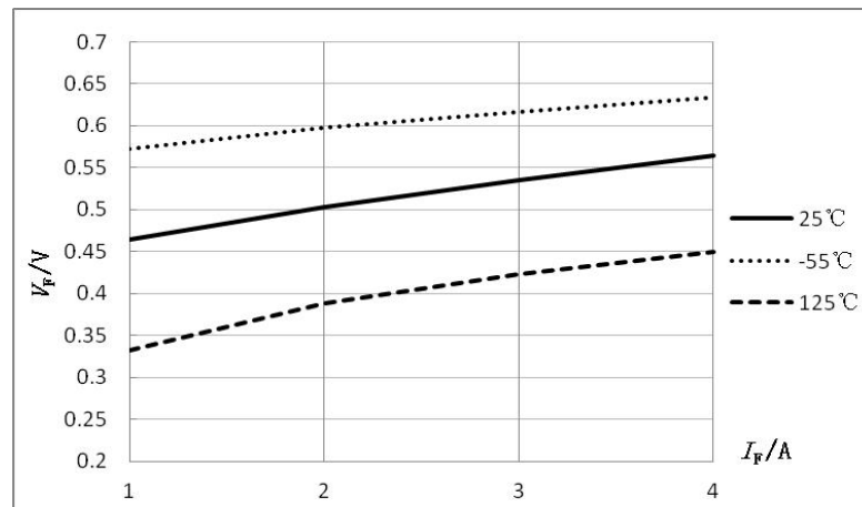
图 2 V_F - I_F 特性曲线
