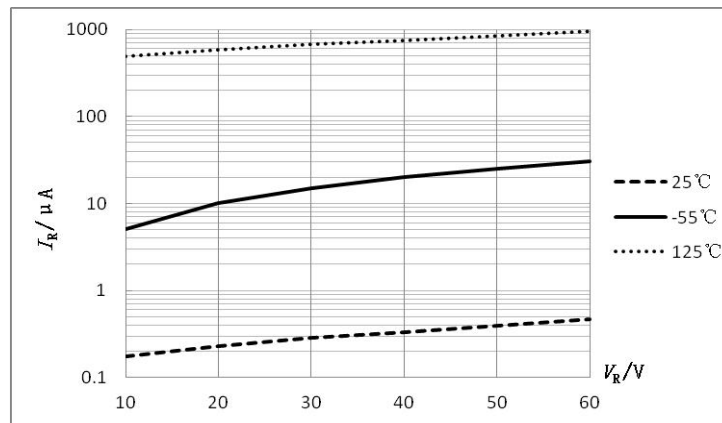
图 1 I_R - V_R 特性曲线
