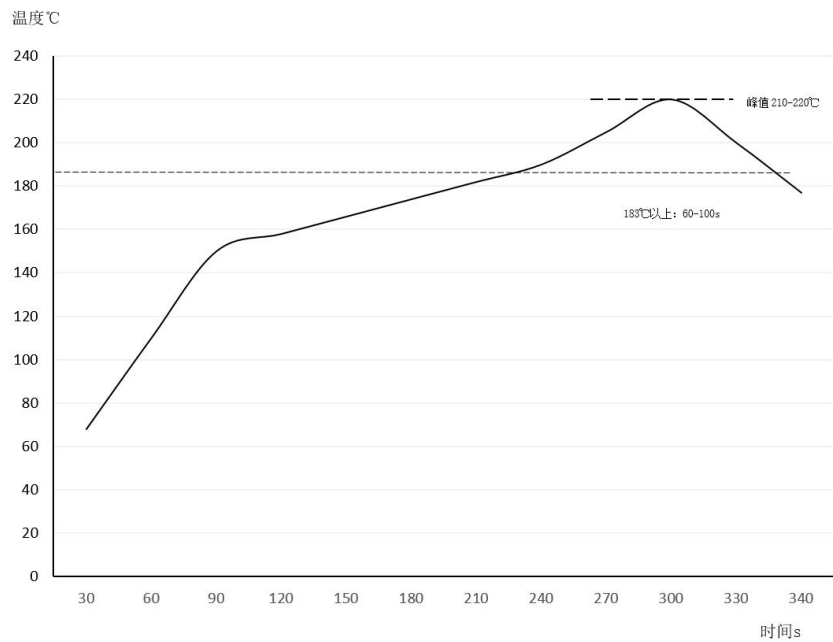
图 7 建议的回流焊曲线
