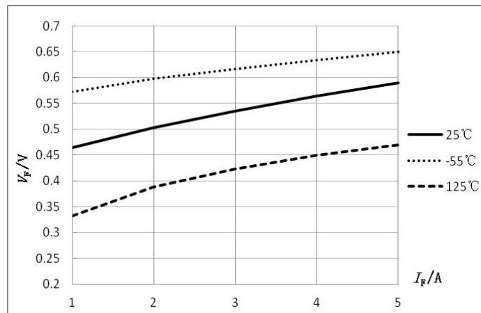
图2 V_F - I_F 特性曲线
