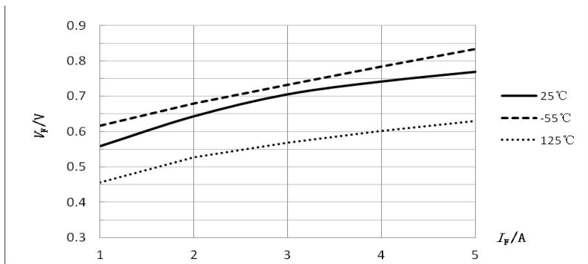
图 2 V_F - I_F 特性曲线
