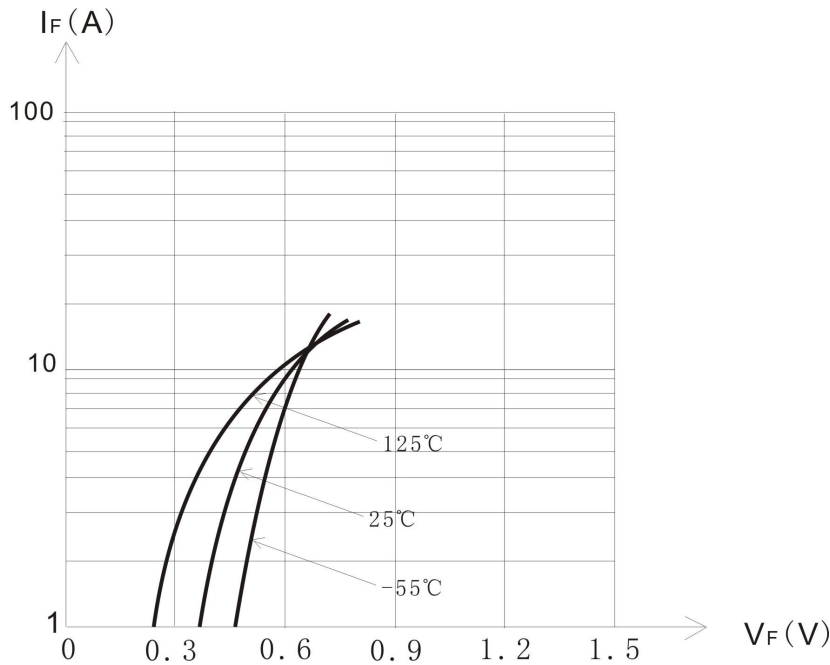
图 2 V_F-I_F 特性曲线
