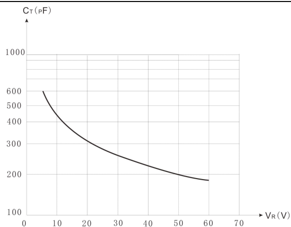
图3 C_T - V_R 特性曲线
