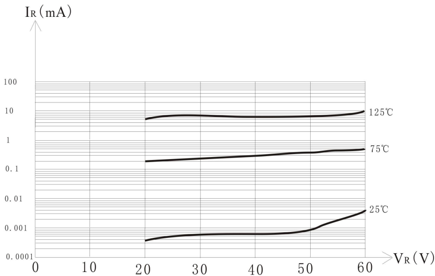
图 1 I_R-V_R 特性曲线
