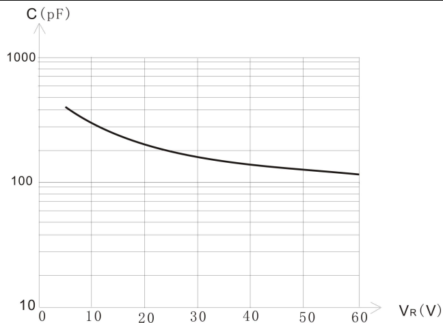
图 3 C_{\text{tot}} — V_R 特性曲线
