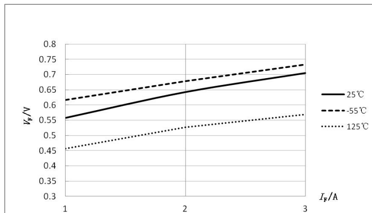
图 2 V_F - I_F 特性曲线
