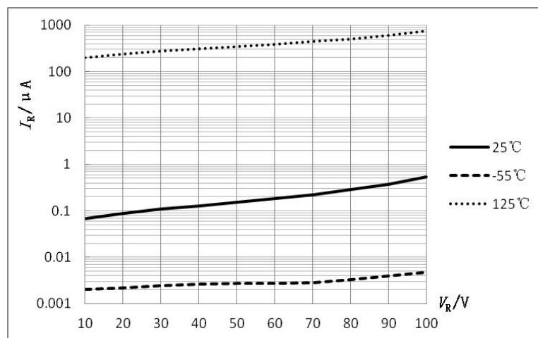
图 1 I_R - V_R 特性曲线
