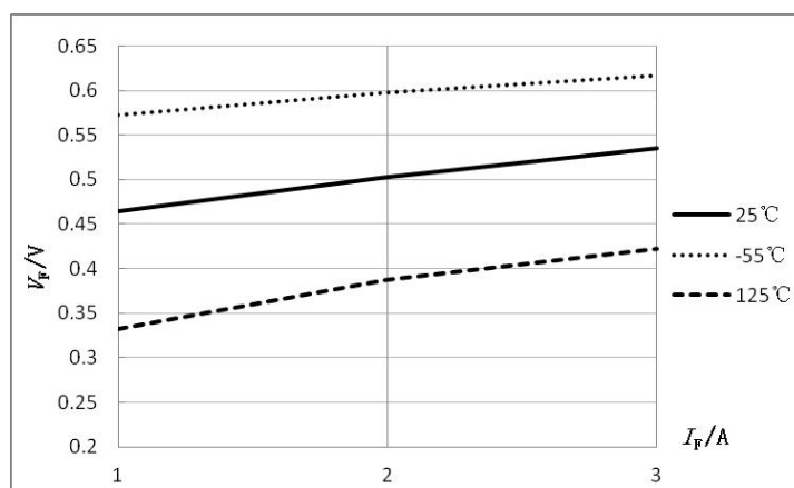
图2 V_F — I_F 特性曲线
