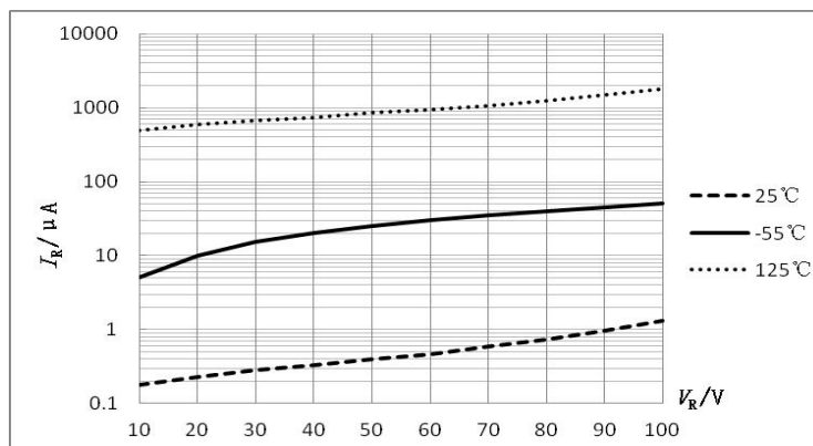
图1 I_R - V_R 特性曲线
