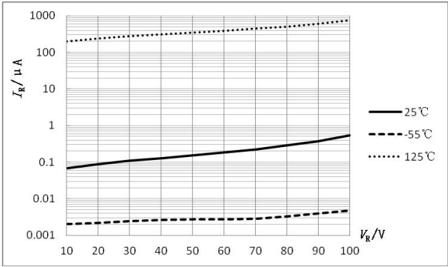
图1 I_R - V_R 特性曲线
