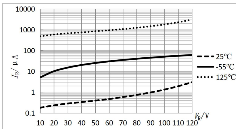
图 1 I_R — V_R 特性曲线
